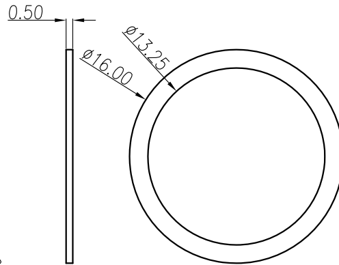
SPACER
