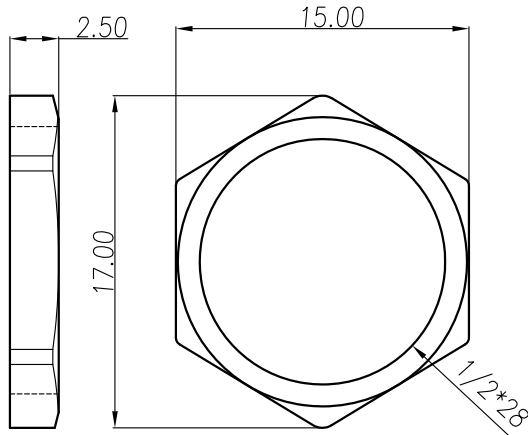
NUT
