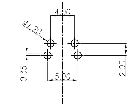
RECOMMEND P.C.B
