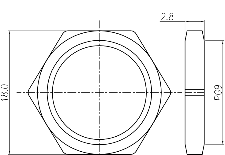
NUT
